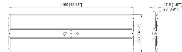
ELSLHB02 4FT 220W / 320W
