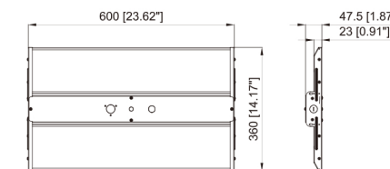
ELSLHB02 2FT 220W
